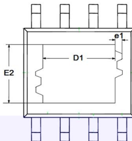
底视图
